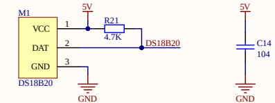
温度传感器模块
