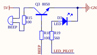
声光报警电路
