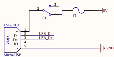
USB电源接口电路
