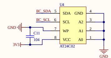
EEPROM存储
