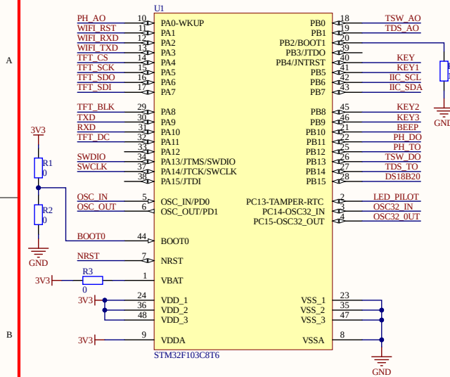
MCU
