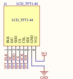
LCD 显示电路
