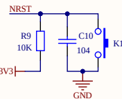
复位电路
