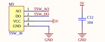
浑浊度传感器模块
