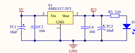
5V - 3V3转换电路
