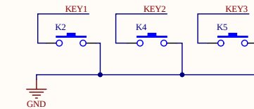
按键电路
