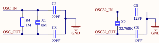
时钟电路
