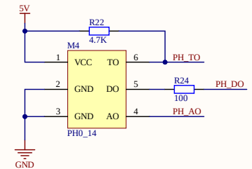
PH传感器模块
